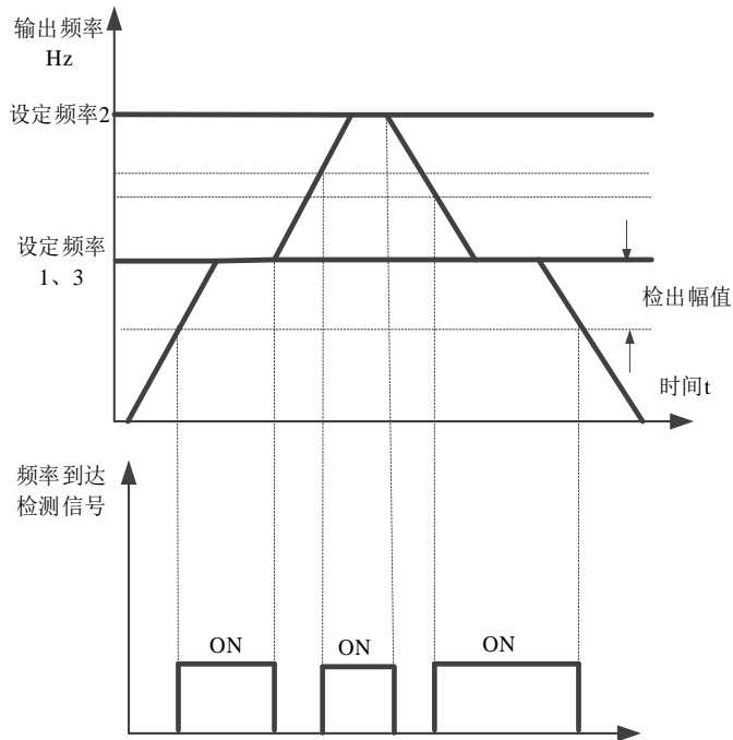
三段速曲线
