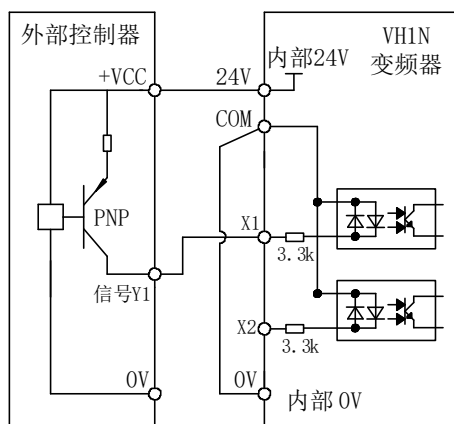
使用变频器内部24V电源的源型接线方法
