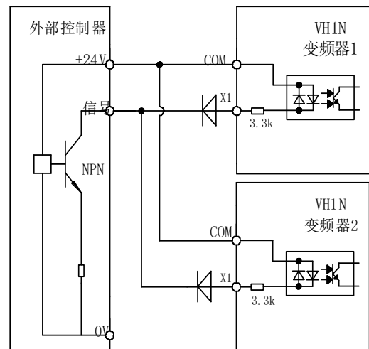
多台变频器使用外部24V电源的漏型接线方法
