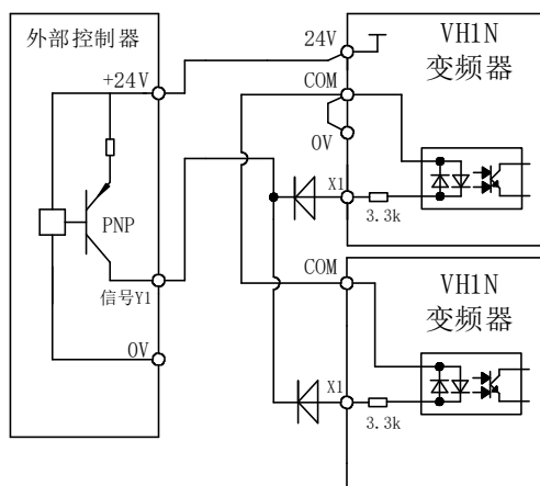
多台变频器使用变频器内部24V电源的源型接线方法
