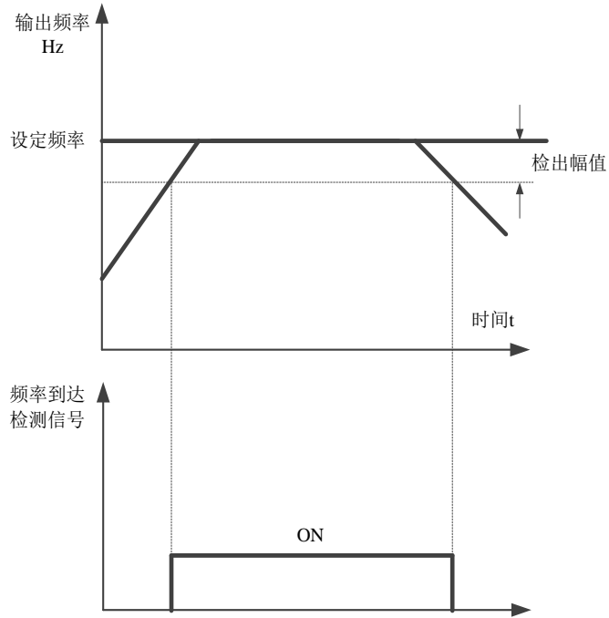
一段速曲线
