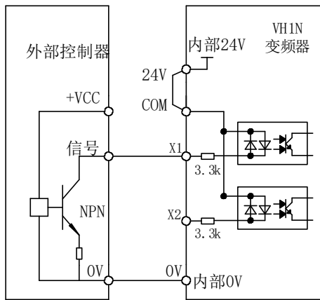
使用变频器内部24V电源的漏型接线方法
